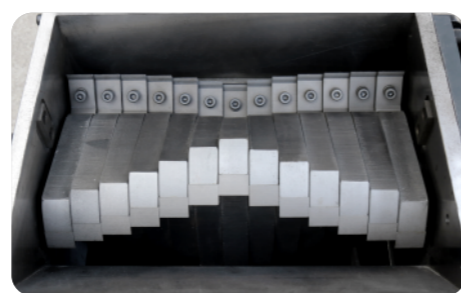
机室 Grinding chamber
